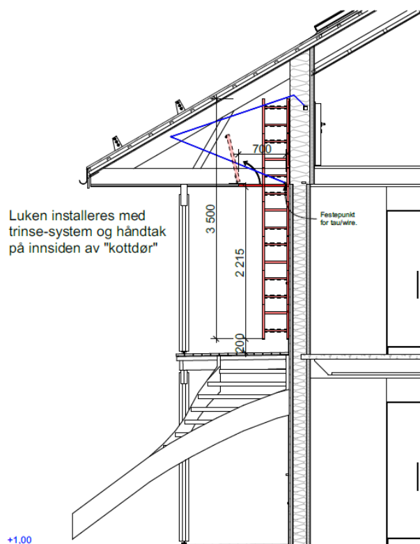
Skisse av luke og stige fra kaldloft
